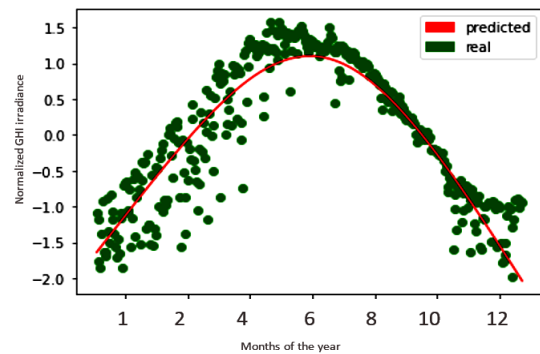
Fig. 14. LSTM output
